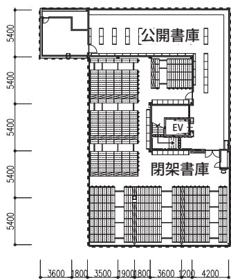
2階平面図
