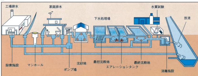
■下水道のしくみ（分流式）
