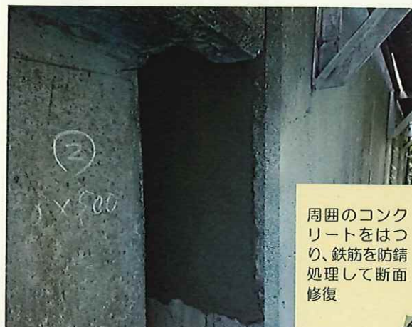
森之腰橋修繕（2018～2019年度）
