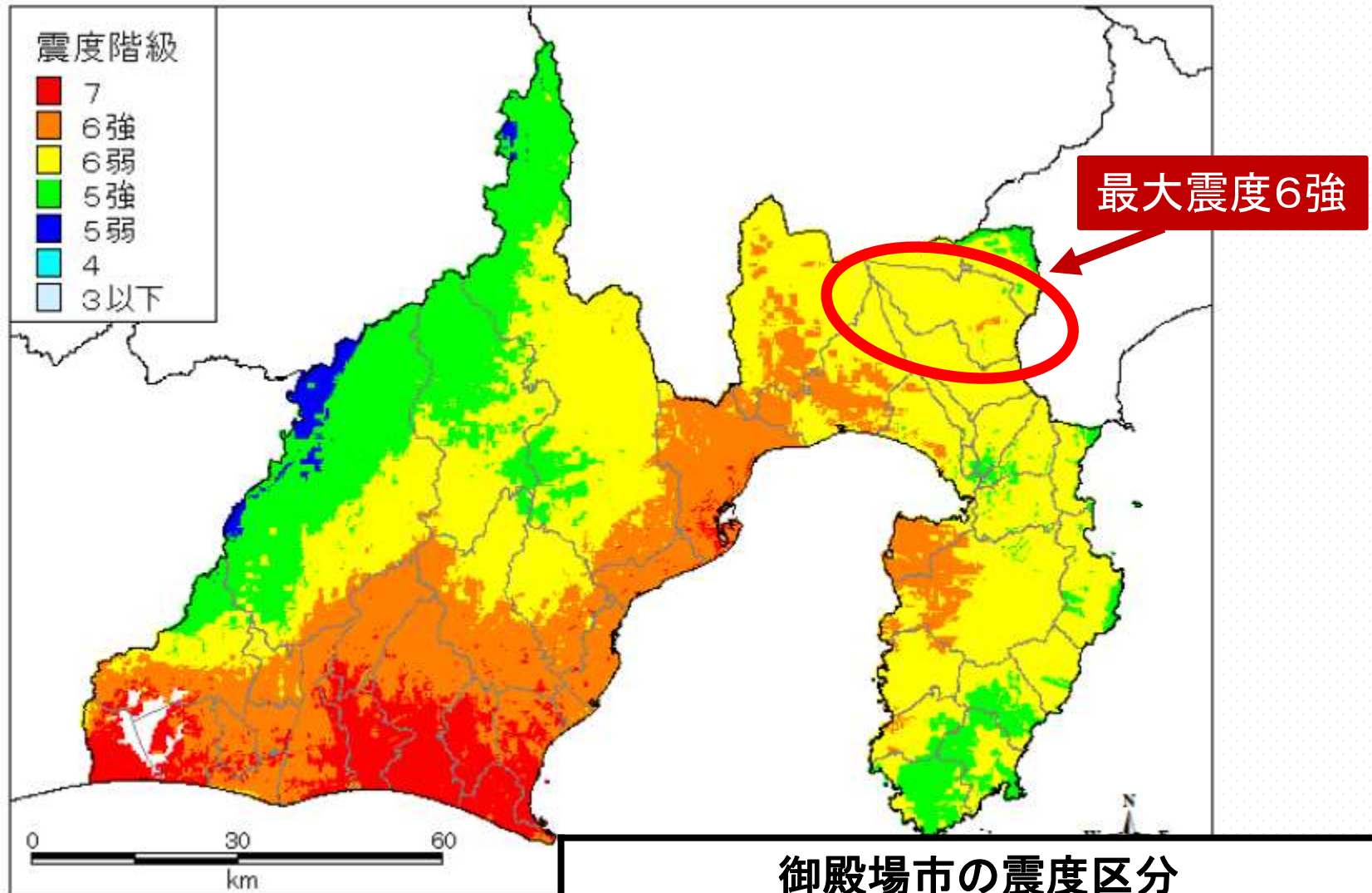
図Ⅱ-1.14 (1) 震度分布図
