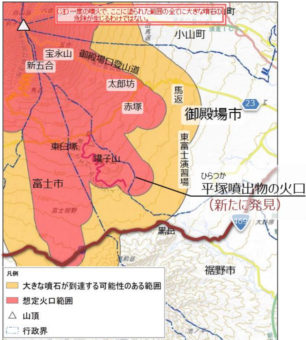
(図2-3) 大きな噴石可能性マップ
